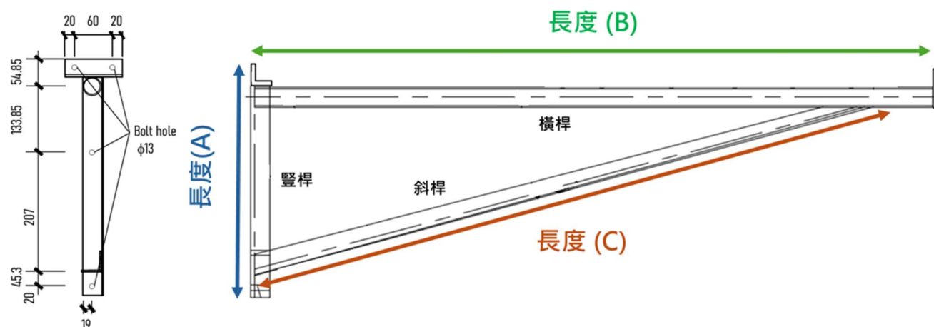
圖二：T 型金屬托架（左架）示意圖（僅供尺寸參考之用）
