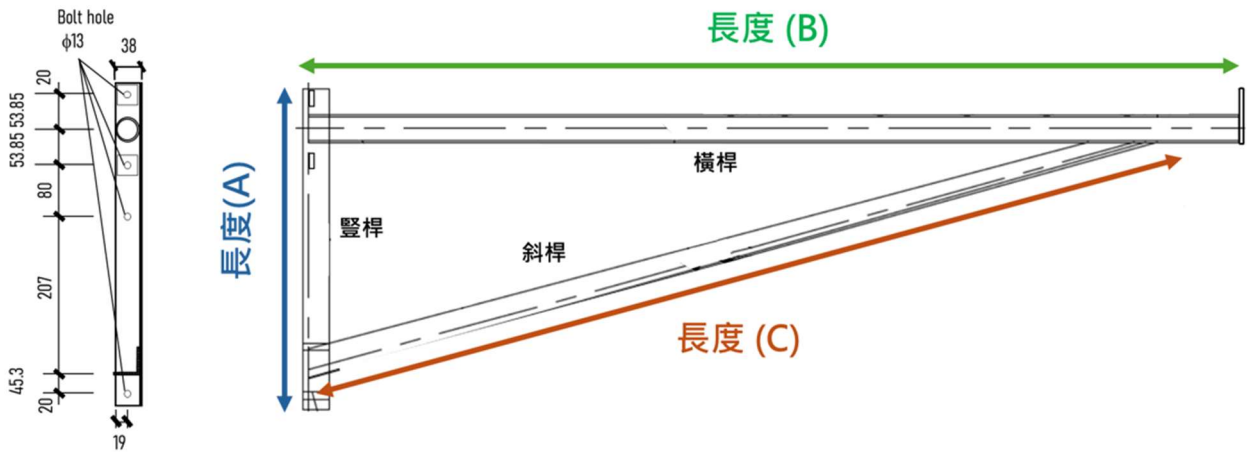
圖一：I 型金屬托架（左架）示意圖（僅供尺寸參考之用）
